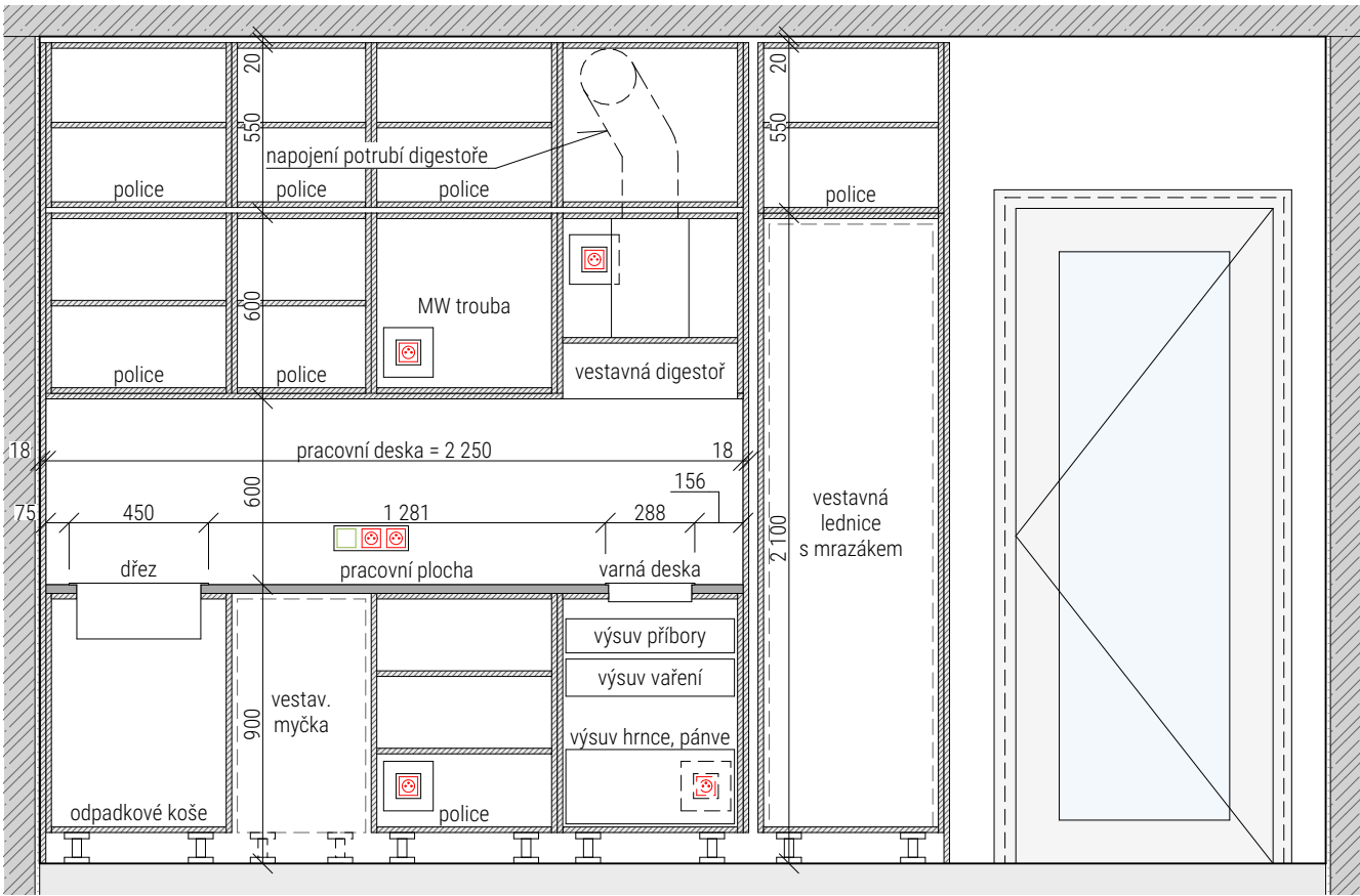
pohled - konstrukce + vybavení
