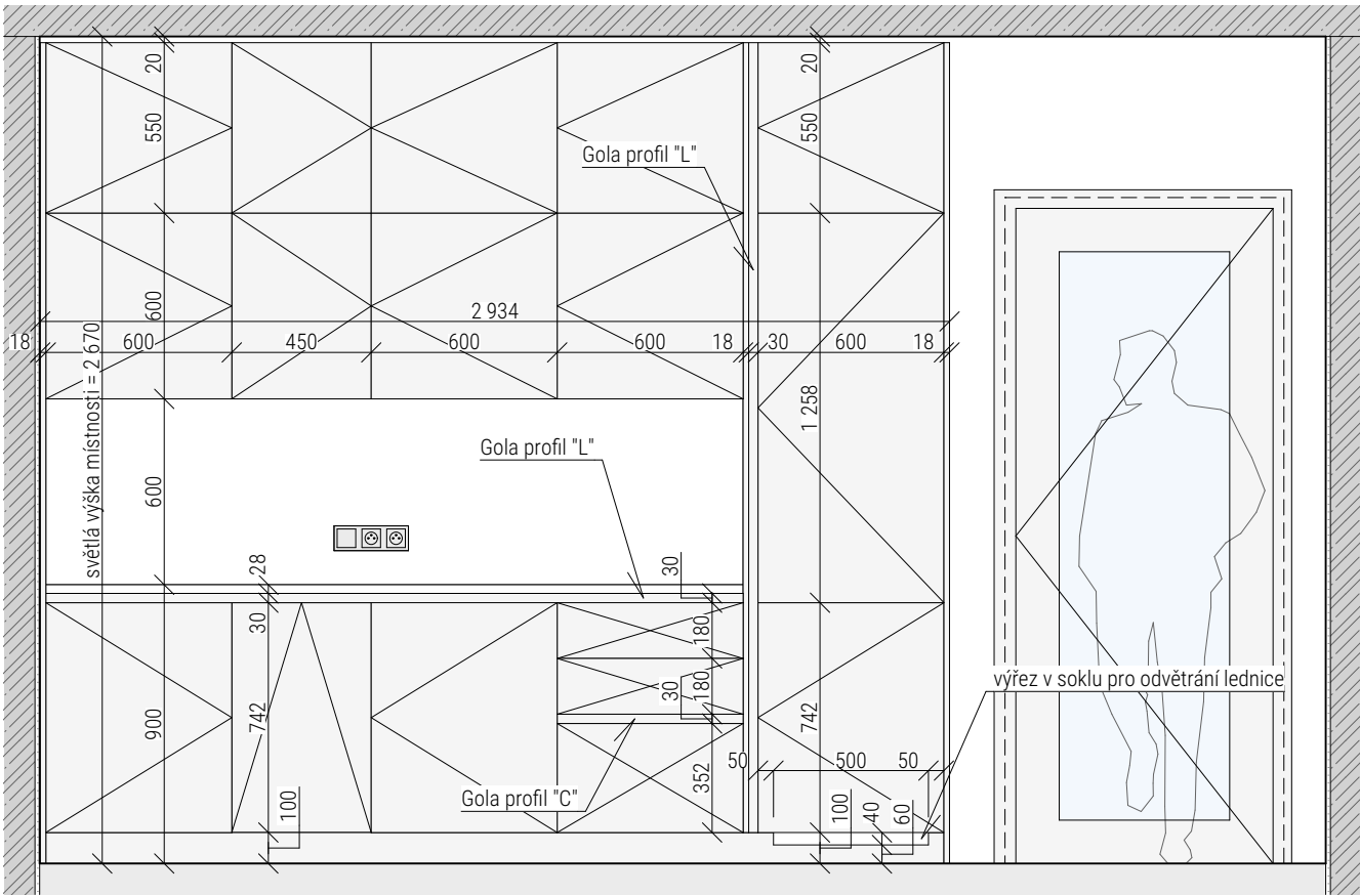
pohled - členění + otevírání
