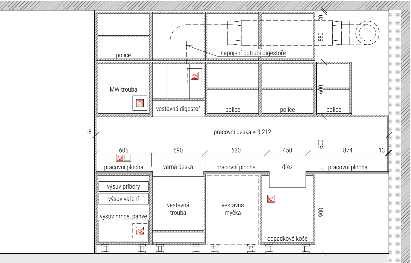
pohled 1 - konstrukce + vybavení
