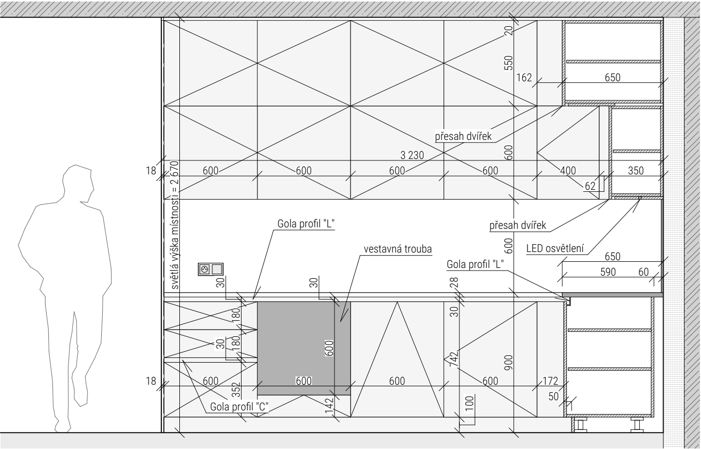
pohled 1 - členění + otevírání
