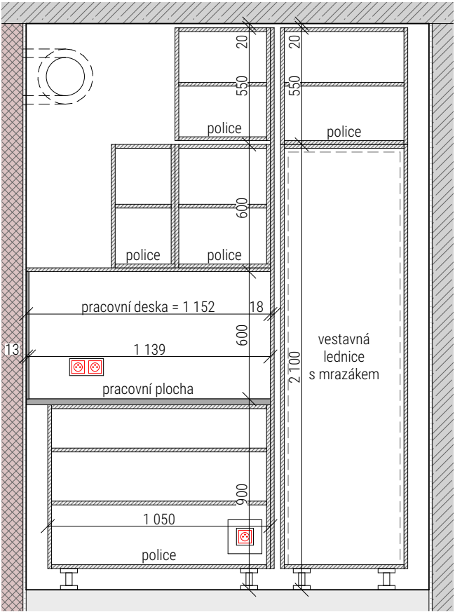
pohled 2 - konstrukce + vybavení
