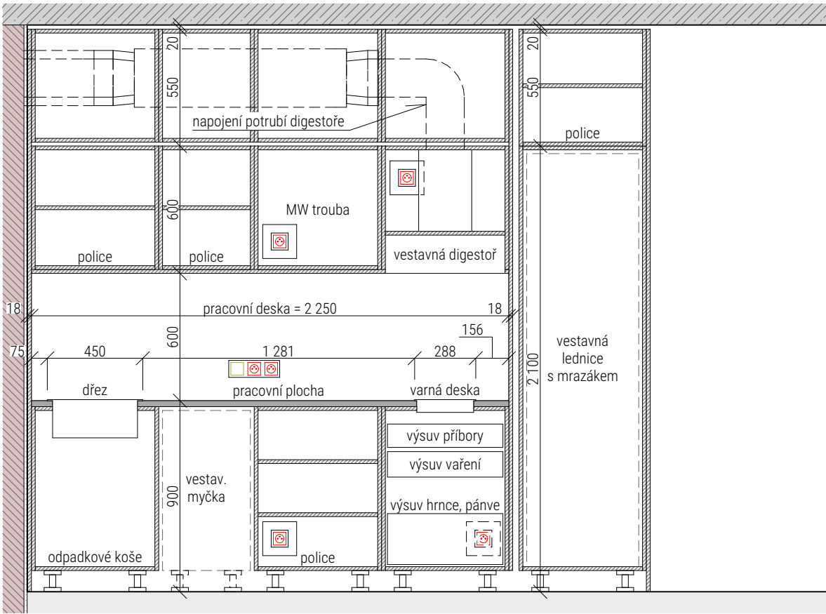
pohled - konstrukce + vybavení
