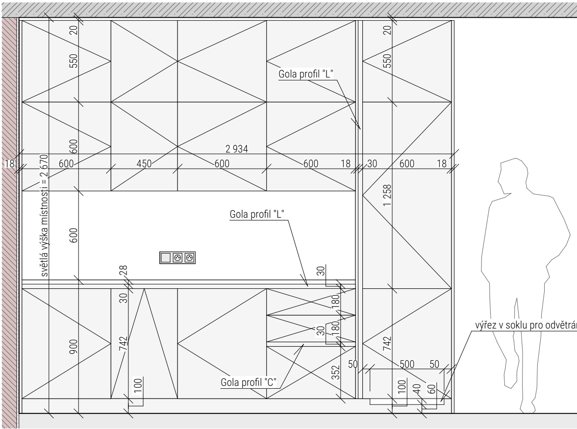
pohled - členění + otevírání
