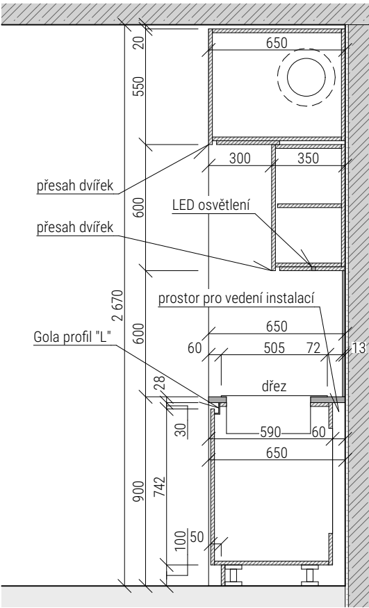
řez - dřezová skříňka
