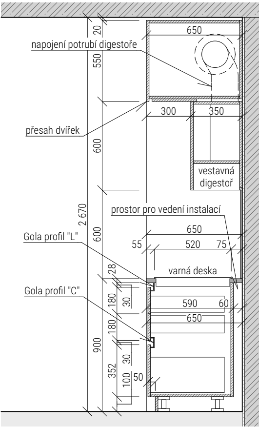
řez - varná deska + digestoř
