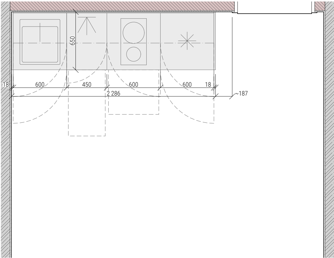
půdorys
